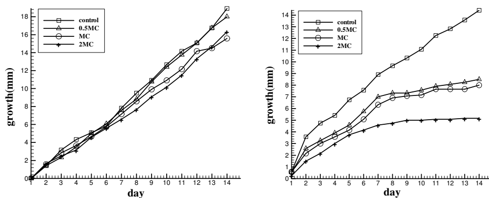
نمودار ۱- اثر غلظت‌های میانگین، نصف غلظت میانگین و دو برابر غلظت میانگین ایمیداکلوپراید روی رشد میسلیم B. bassiana (چپ) و L. muscarium (راست) Fig. 1. Effect of concentrations MC, 1/2 MC and 2 MC on mycelium growth of Beauveria bassiana (Left) and Lecanicillium muscarium (right)
